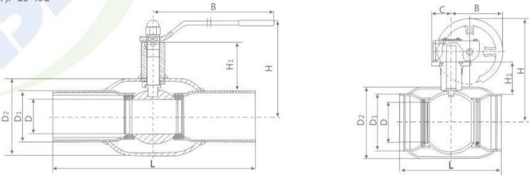
结构图Structure diagram QW(3)4(6)1(7)F-16-40C
