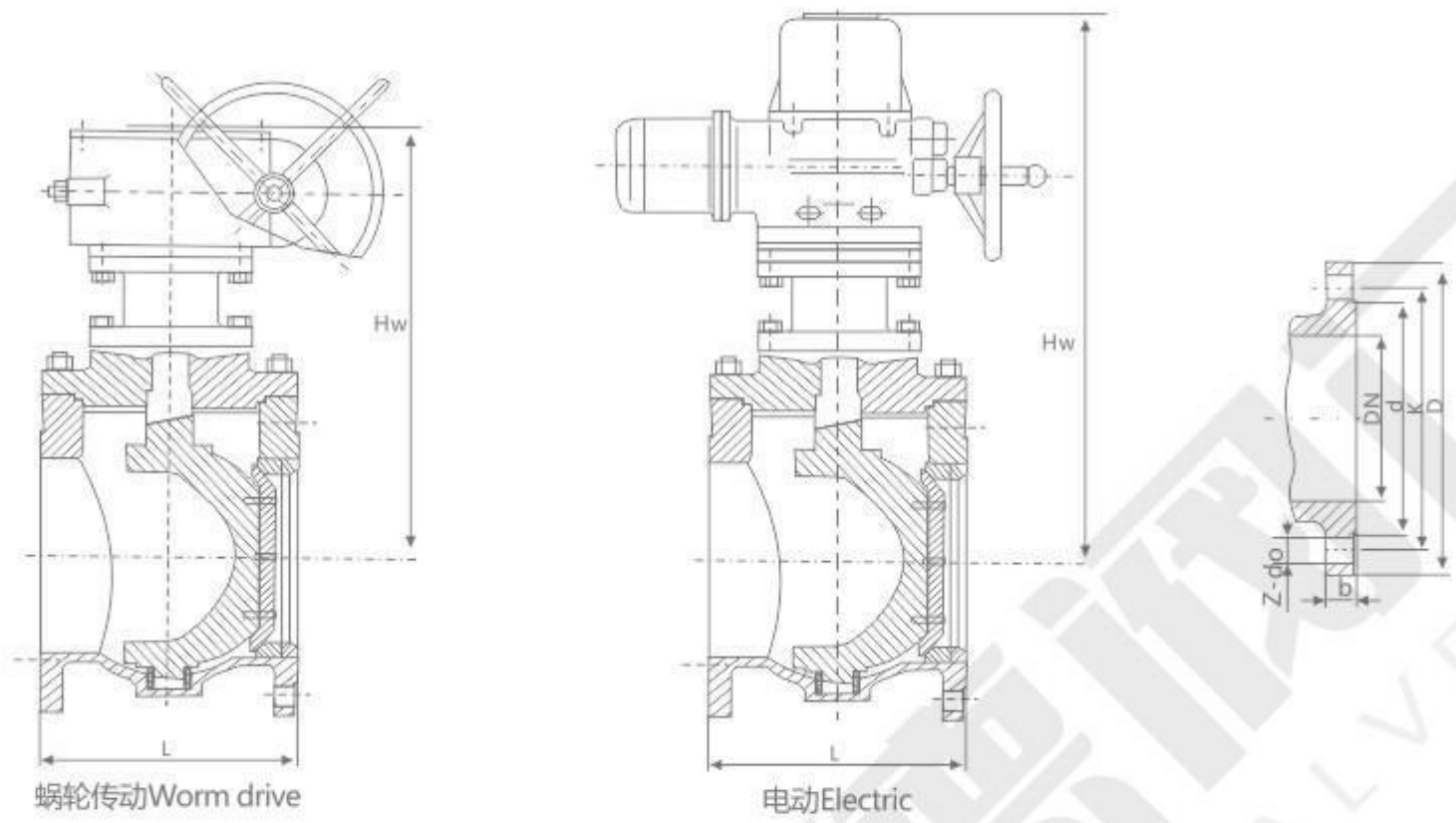
主要连接尺寸 Main connection dimensions
