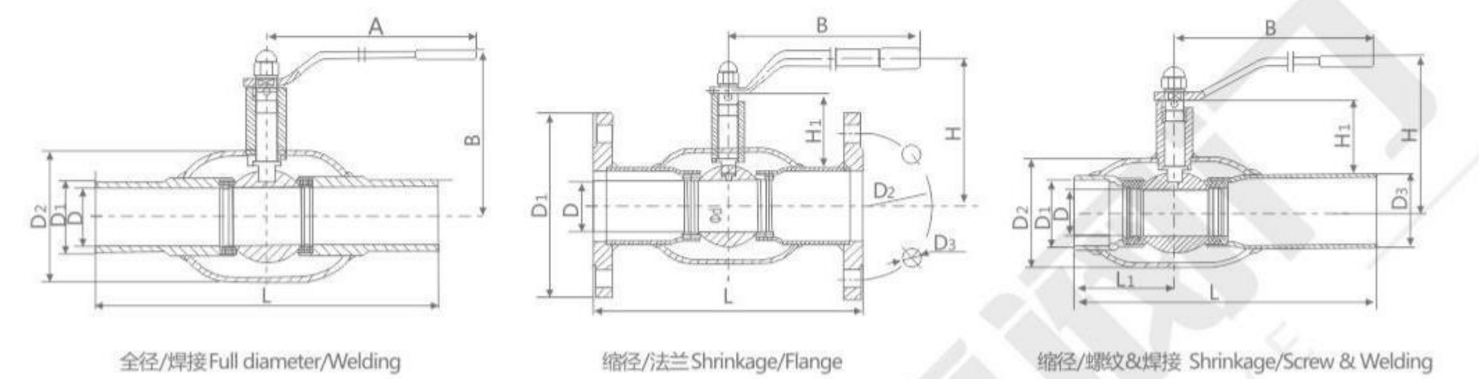
结构图Structure diagram QW(3)4(6)1(7)F-16-40C
